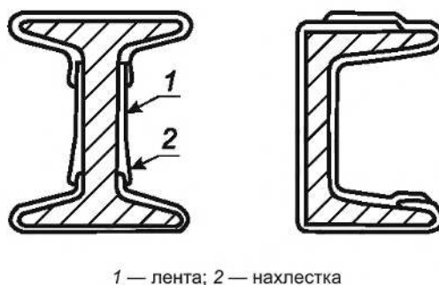
Рисунок Е.11 — Примеры изоляции поверхности профилей пластиковыми лентами
