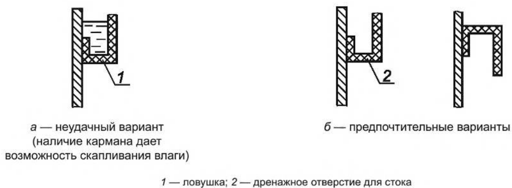
Рисунок Е.5 — Примеры устранения возможности скапливания влаги
