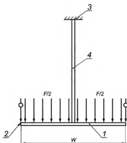
1 — кронштейн с центральной опорой; 2 — точка измерения прогиба на конце кронштейна с центральной опорой; 3 — жесткая конструкция; 4 — подвес; F/2 — нагрузка на кронштейн с каждой стороны подвеса; W — длина кронштейна с центральной опорой
