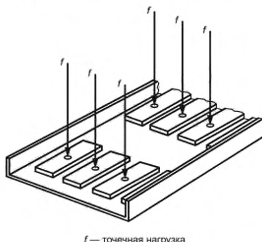
Рисунок D.2 — Типичное расположение пластин распределения нагрузки
