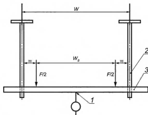
1 — точка измерения прогиба на середине между; 2 — подвес; 3 — трапециевидная опора; F — сила на трапециевидную опору; W — ширина между осями подвесов; W_s — расстояние между средними линиями контактных участков
