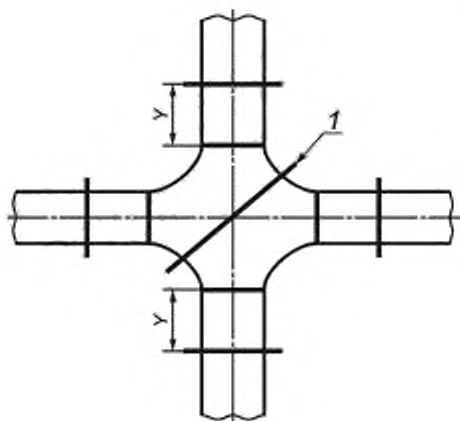
Рисунок 17 — Испытание безопасной рабочей нагрузки для горизонтальной равносторонней крестообразной секции
