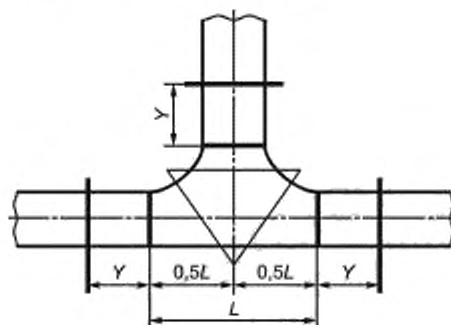
Рисунок 16 — Испытание безопасной рабочей нагрузки для горизонтальной равносторонней Т-образной секции
