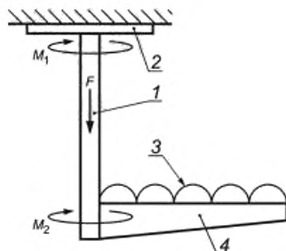
1 — подвес; 2 — основание подвеса; 3 — нагрузка на консольный кронштейн; 4 — консольный кронштейн; F — сила вырывания подвеса; M_1 — изгибающий момент на потолочной плите; M_2 — изгибающий момент от консольного кронштейна
