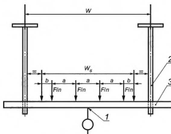
1 — точка измерения прогиба на середине между подвесами; 2 — подвес; 3 — трапециевидная опора; a - a = W_s/n ; b - b = a/2 ; F — сила РРН на трапециевидную опору, n — количество точечных нагрузок согласно приложению D; W — ширина между осевыми линиями подвеса; W_s — ширина кабельного лотка/лестницы
