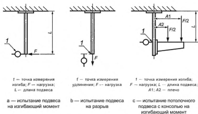
Рисунок 21 — Испытание подвеса
