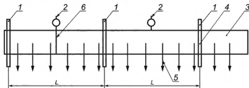
1 — жесткая опора для кабельного лотка; 2 — измерения прогиба (см. рисунок 10); 3 — кабельный лоток; 4 — место фиксации лотка к опорам; 5 — нагрузка; 6 — стык кабельных лотков; L — расстояние между пролетами опор
