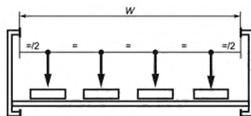
Рисунок D.1 — Примеры точек распределения нагрузки по ширине
