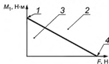
1 — БРН по 10.8.2.1 (для подвеса в соответствии с рисунком 21а); 2 — опасная область; 3 — область безопасных нагрузок; 4 — БРН по 10.8.2.2 (для подвеса в соответствии с рисунком 21б)
