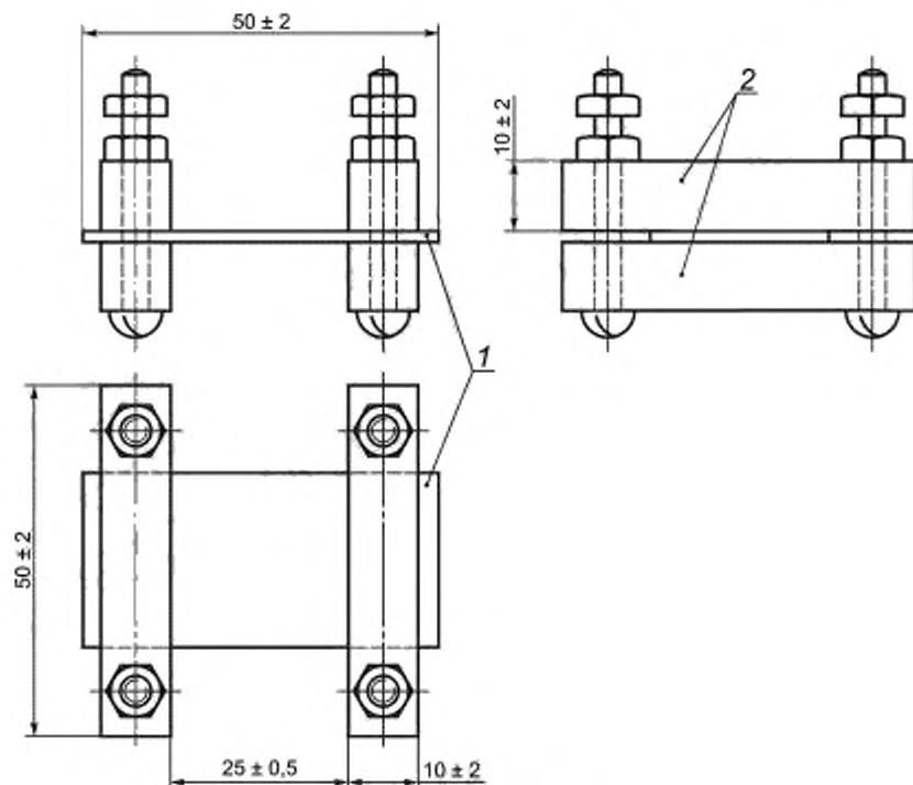
1 — образец; 2 — электроды
