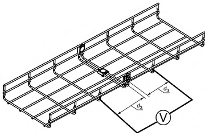
в — сопротивление стыка проволочного лотка с отдельным соединителем
