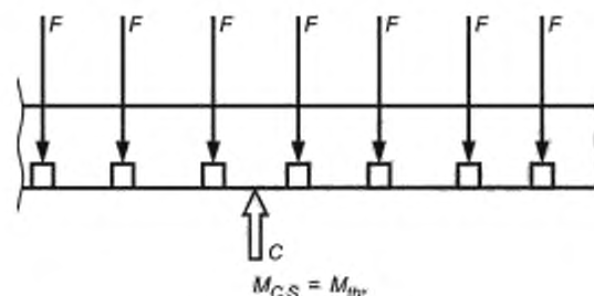
Рисунок D.5 — Пример консольно-закрепленного участка с четырьмя и более перемычками
