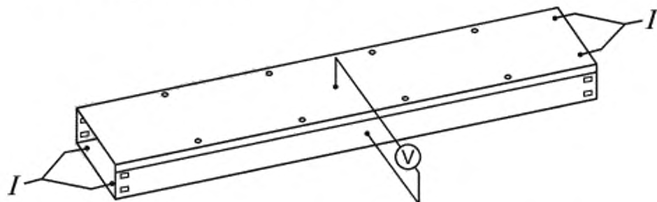
Рисунок 31 — Схема проведения испытания на сопротивление соединения между крышкой доступа и кабельным лотком или кабельной лестницей
