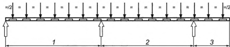
1 — конечный пролет длиной L или X , указанной изготовителем; 2 — промежуточный пролет длиной L ; 3 — консольно-закрепленный участок длиной 0,4L
