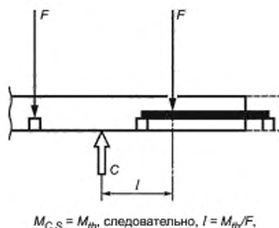
Рисунок D.9 — Пример приложения нагрузки на консольно-закрепленном участке с наращиванием длины участка
